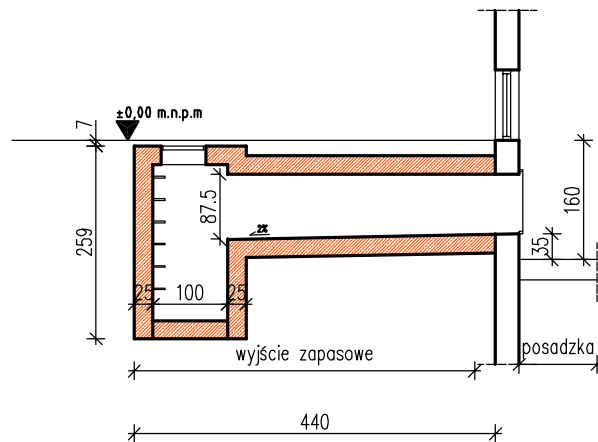
PRZEKRÓJ A-A
