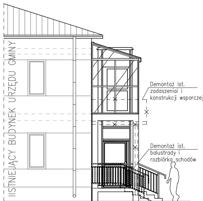
ELEWACJA POŁUDNIOWA
