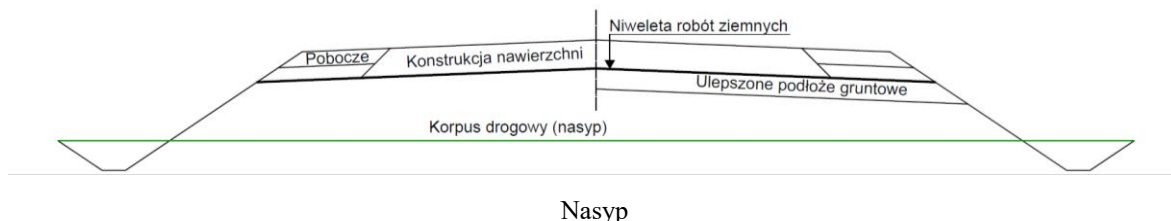
Rysunek 1.1. Lokalizacja niwelety robót ziemnych
