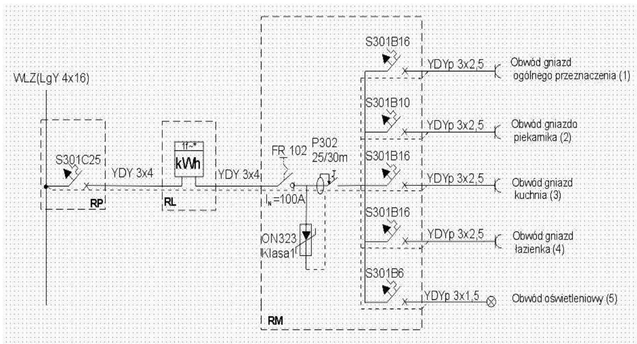
Rys. 1. Przykładowy schemat jednokreskowy instalacji elektrycznej w lokalu mieszkalnym
