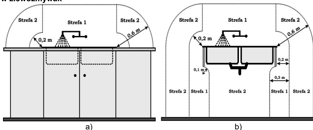
Rys. 3. Strefy w pomieszczeniach wyposażonych w zlewozmywak a) zabudowany, b) niezabudowany.
