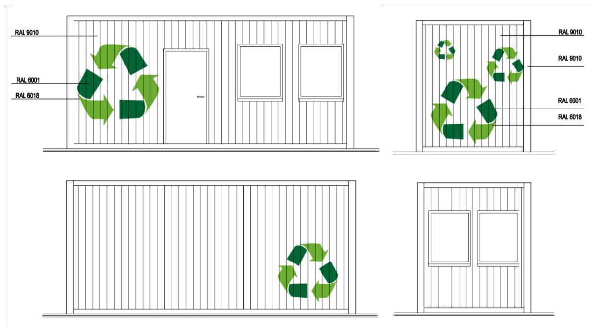
Ryc. 8. Kontener socjalno biurowy – elewacje
