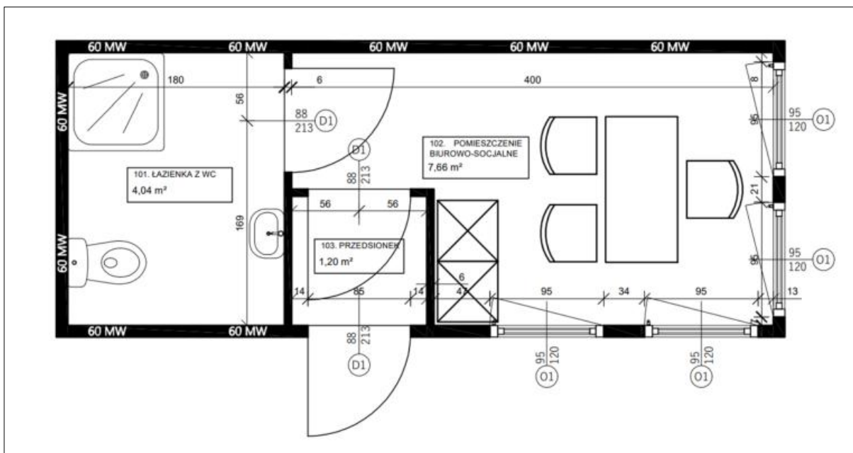
Ryc. 7. Kontener socjalno biurowy – rzut ze schematem wyposażenia (przykład poglądowy, do dostosowania do wymogów prawnych)
