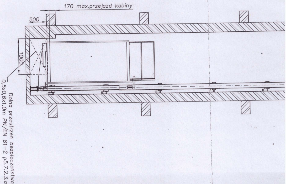
Rys.1 Przekroj pionowy szybu
