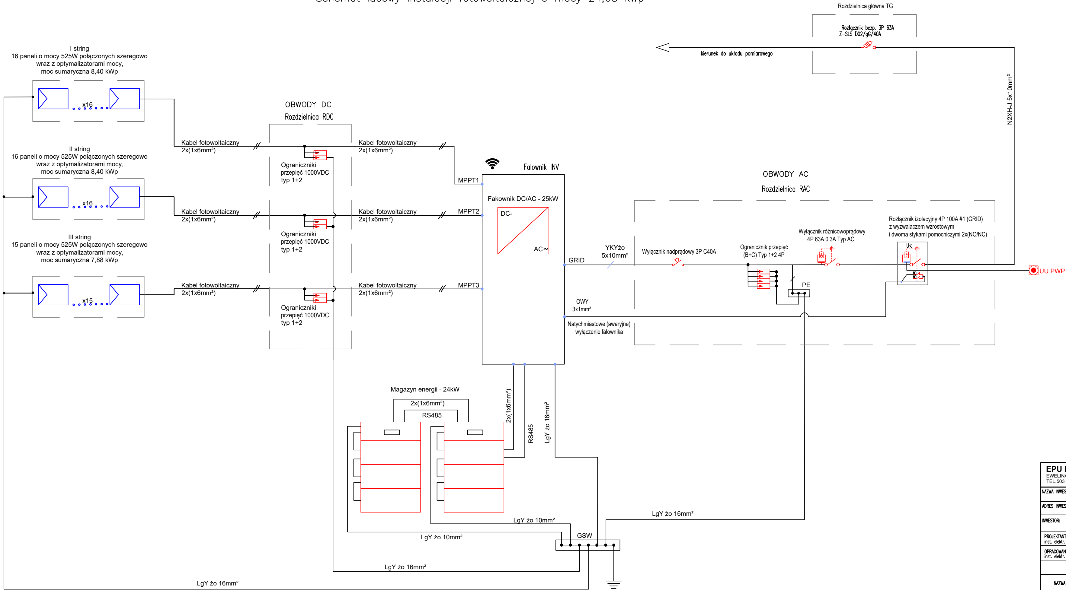
Schemat ideowy instalacji fotowoltaicznej o mocy 24,68 kWp
