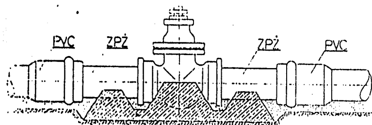
Blok podporowy dla zasuwy żeliwnej
