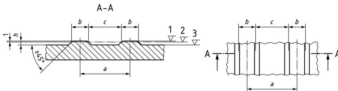
Rys. 1a. Płytki kierunkowa symetryczna - prowadząca- szczegół powierzchni
