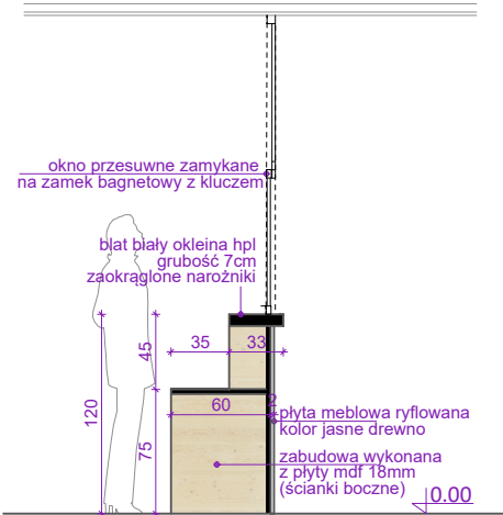
widok boczny lady recepcyjnej
