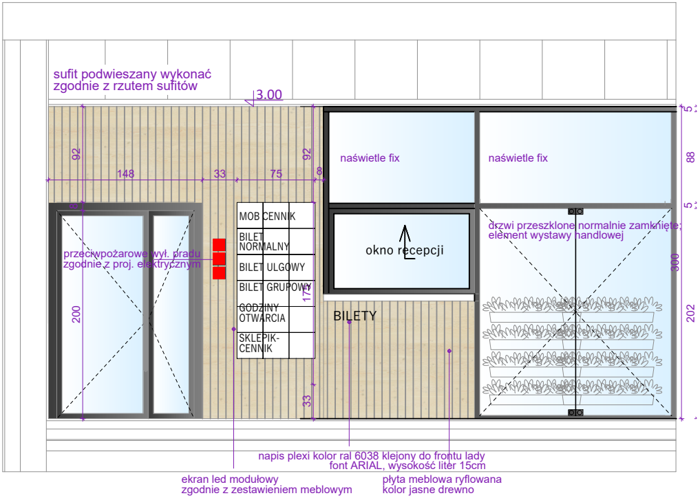
rozwińnięcie ściany wejściowej
