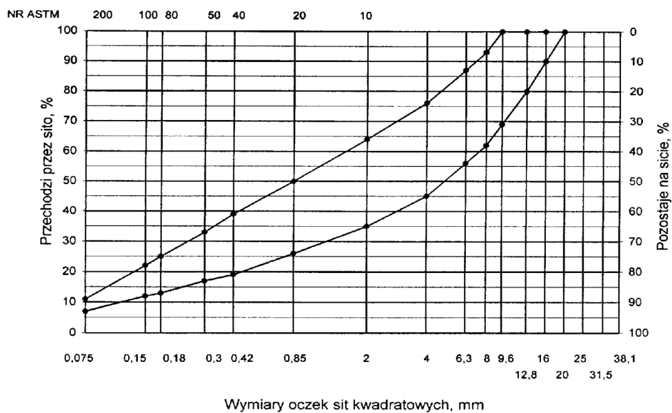
Rys. 2. Krzywe graniczne
