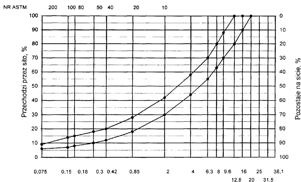
Rys. 6. Krzywe graniczne uziarnienia mieszanki mineralnej BA od 0 do 16 mm do warstwy ścieralnej
