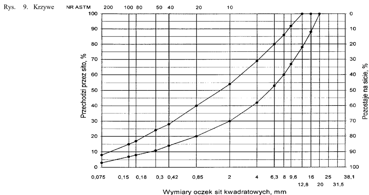
graniczne uziarnienia mieszanki mineralnej BA od 0 do 16 mm do warstwy wiążącej, wyrównawczej i wzmacniającej nawierzchni drogi o obciążeniu ruchem KR1 lub KR2
