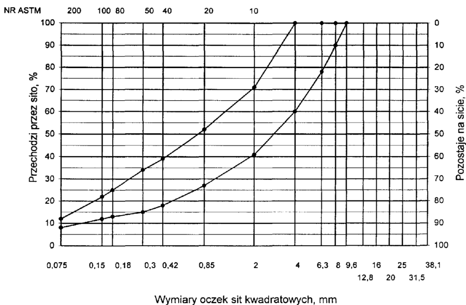
Rys. 3. Krzywe graniczne uziarnienia mieszanki mineralnej BA od 0 do 16mm, od 0 do 12,8 mm do warstwy ścieralnej nawierzchni drogi o obciążeniu ruchem KR1 lub KR2 6,3 mm do warstwy ścieralnej nawierzchni drogi o obciążeniu ruchem nawierzchni drogi o obciążeniu ruchem KR1 lub KR2
