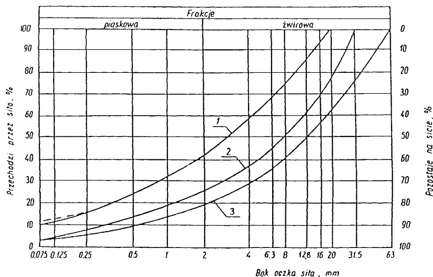
Rysunek 1. Pole dobrego uziarnienia kruszyw przeznaczonych na podbudowy wykonywane metodą stabilizacji mechanicznej 1-2 kruszywo na podbudowę
