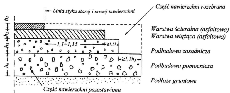
Rys. 2. Konstrukcja połączenia starej i nowej nawierzchni
